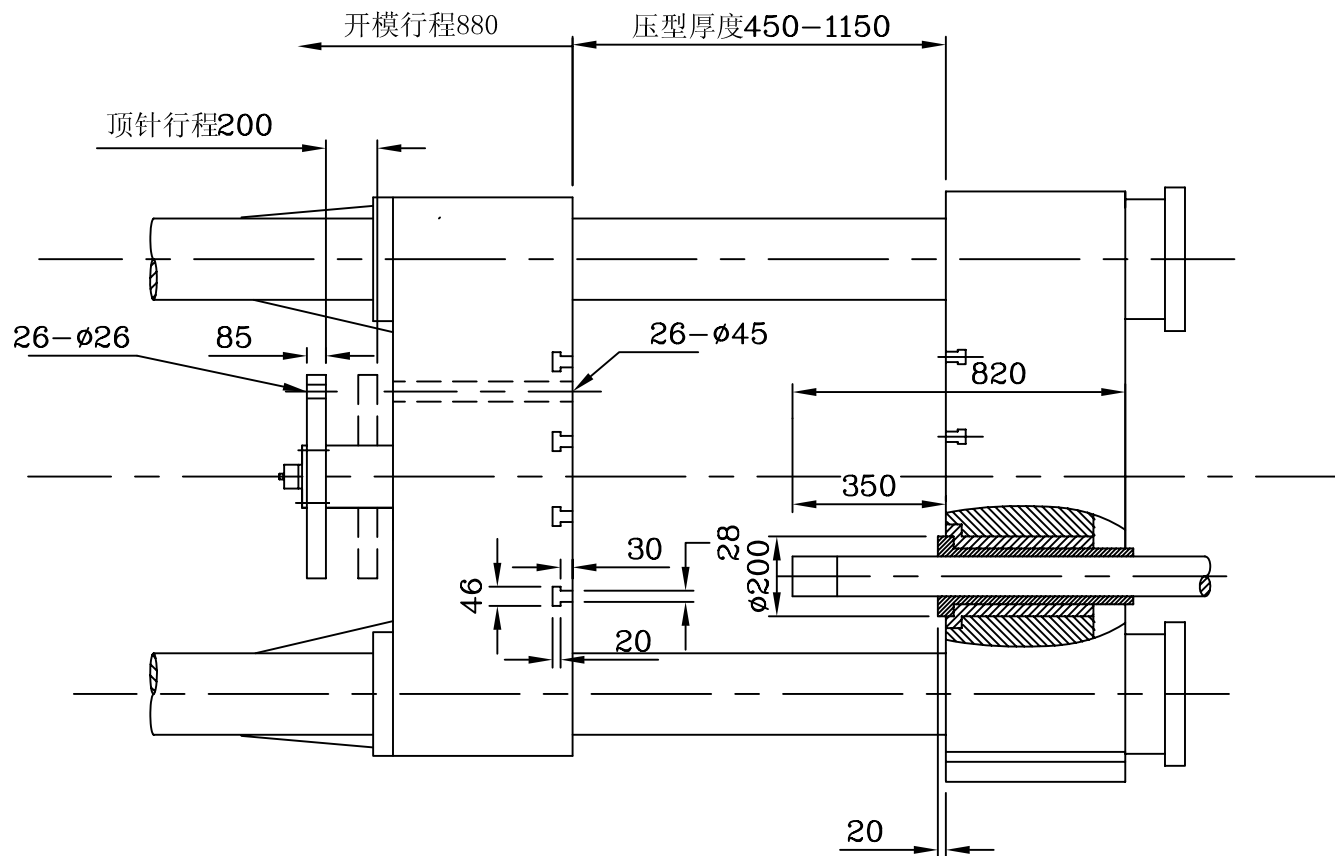
NX1000C 模板尺寸图
