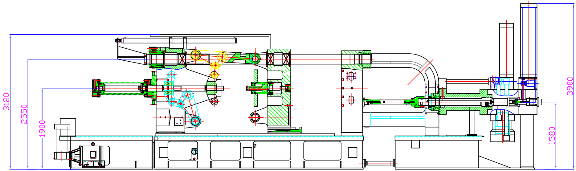
上海三基 DC1250C外形图
