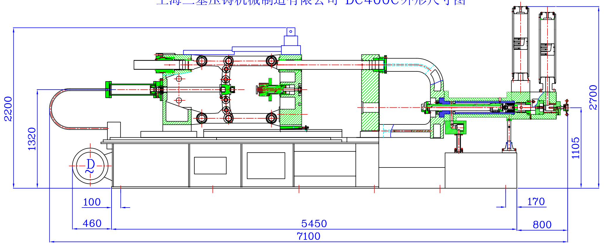
上海三基压铸机械制造有限公司 DC400C外形尺寸图
