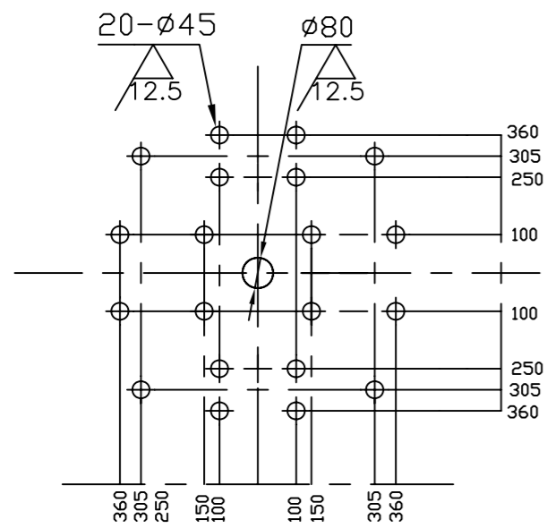
顶针孔位图
