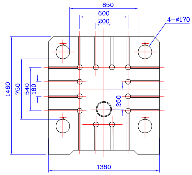
DC-700C 模板图尺寸图
