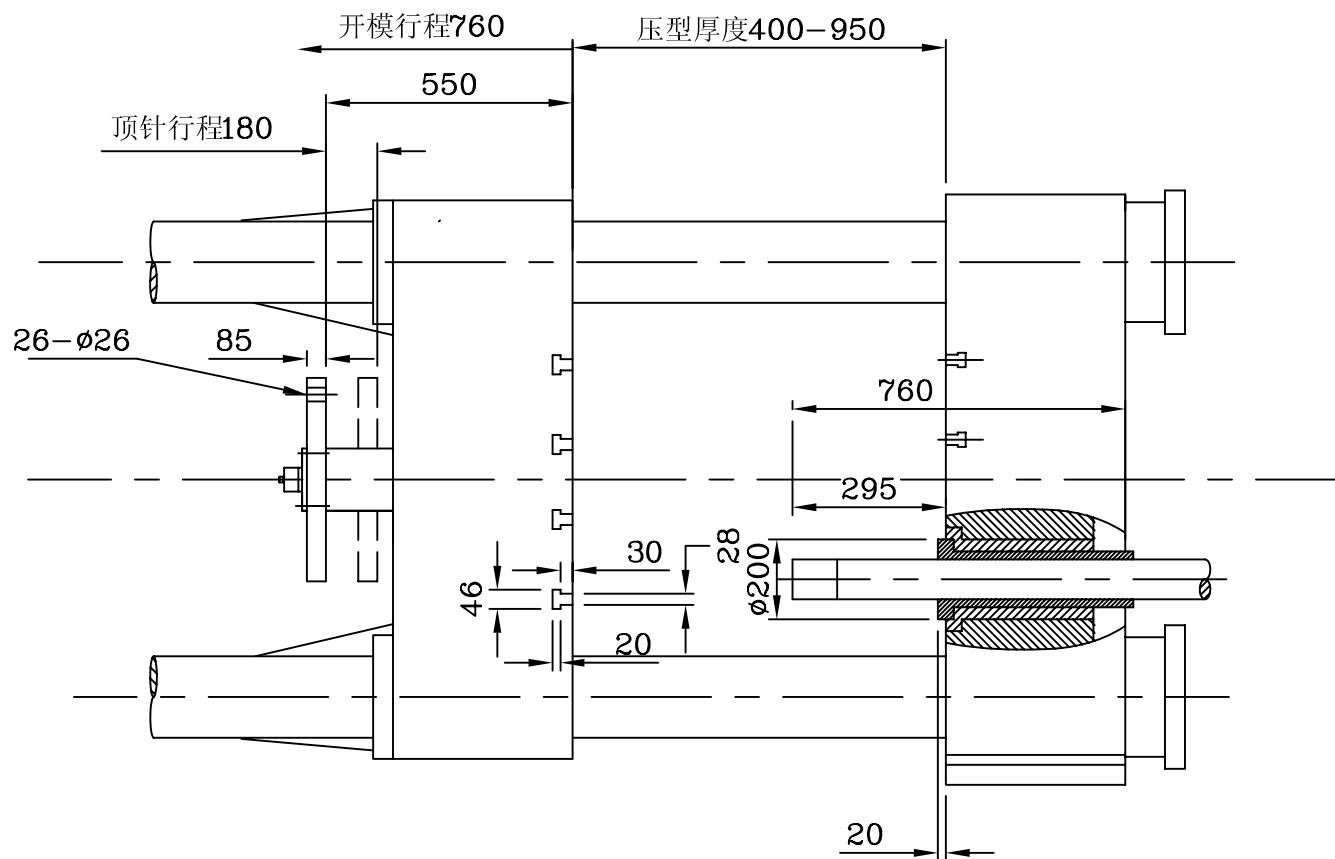
DC800C 模板尺寸图
